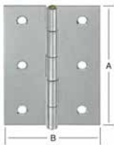
Gerold halfbrede verzinkte scharnieren DIN 7954 B met vaste messing stift
