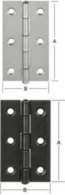
Gerold smalle scharnieren DIN7954A met vaste messing stift
