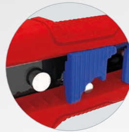
Trekvaste mesvergrendeling en mesborgen van gehard staal
