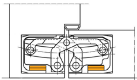
Doorsnede TECTUS FR
